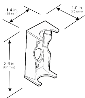
Support de montage pour SU- 5E
